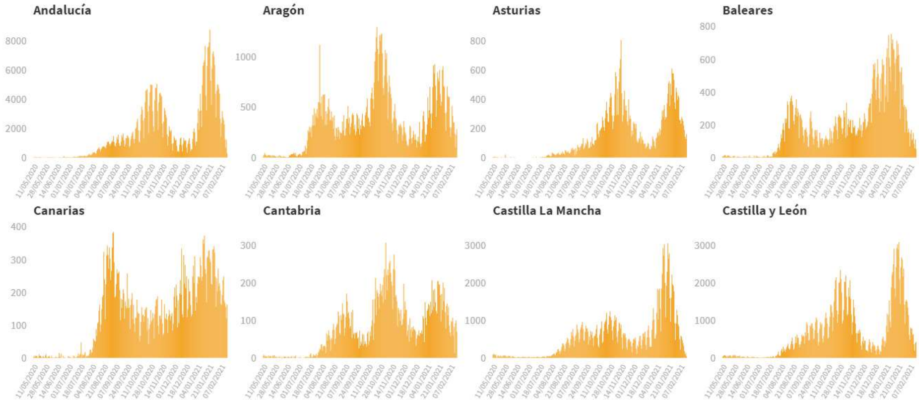
Figura 3. Casos diarios confirmados de COVID-19 por fecha de diagnóstico desde el 11.05.2020 por Comunidades Autónomas, a 16.02.2021 (datos consolidados a las 14:00 horas del 17.02.2021).
