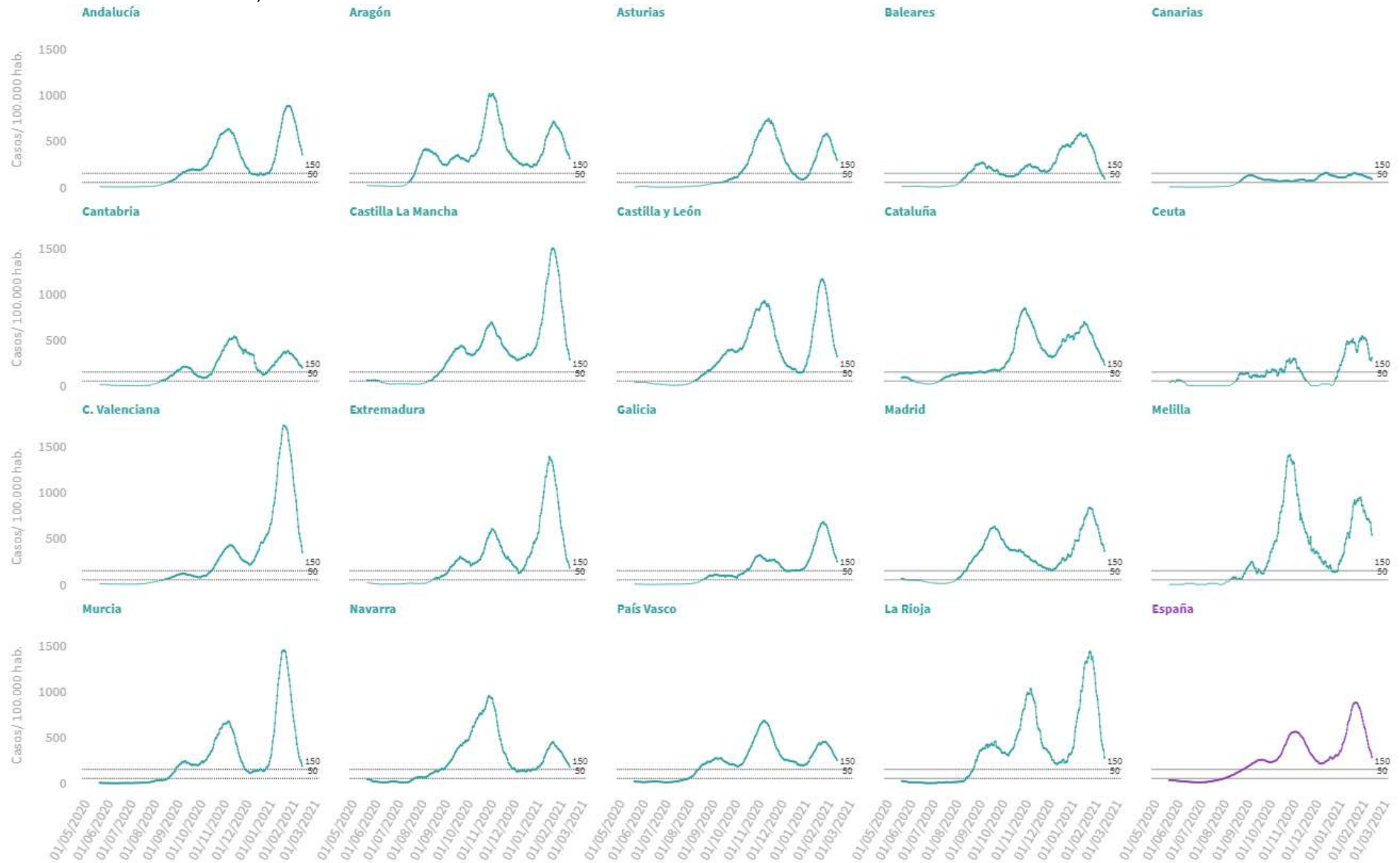
Figura 6. Incidencia acumulada en 14 días en mayores de 64 años por fecha de diagnóstico desde el 11.05.2020 por Comunidades Autónomas, a 16.02.2021 (datos consolidados a las 14:00 horas del 17.02.2021).
